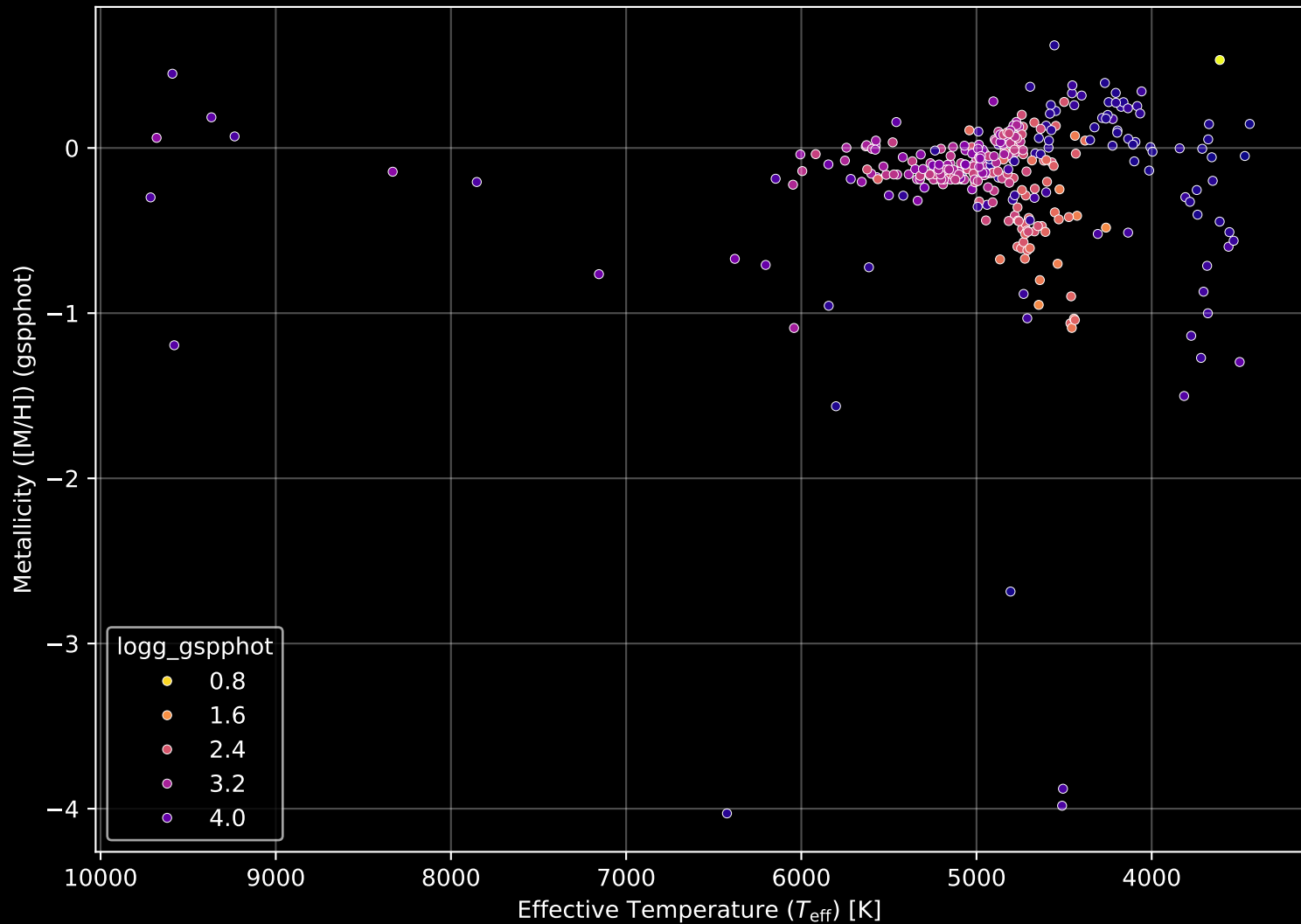
APOGEE DR17 Field: [155-27_btx] Stellar Population Parameters (n= 322)
